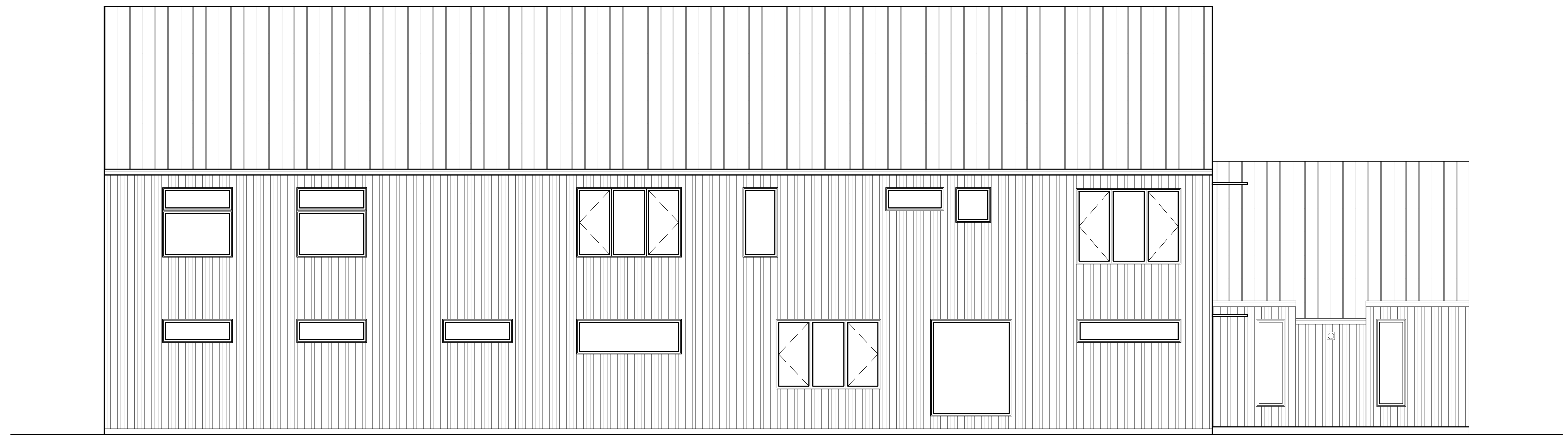
RIGHT ELEVATION
