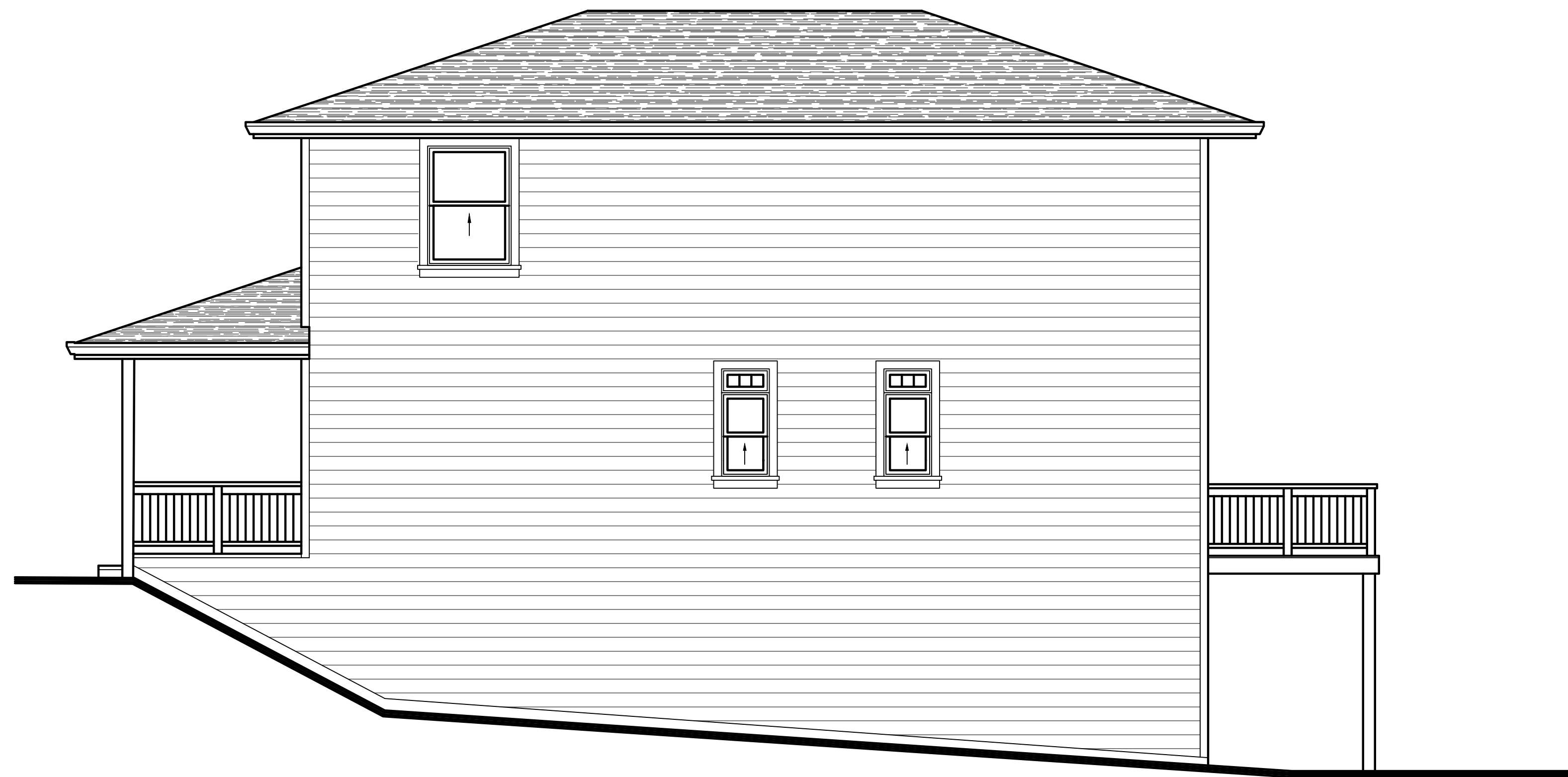
RIGHT ELEVATION
