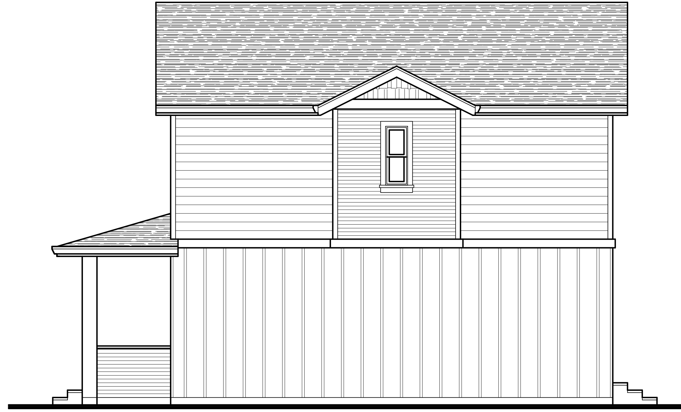
RIGHT ELEVATION
